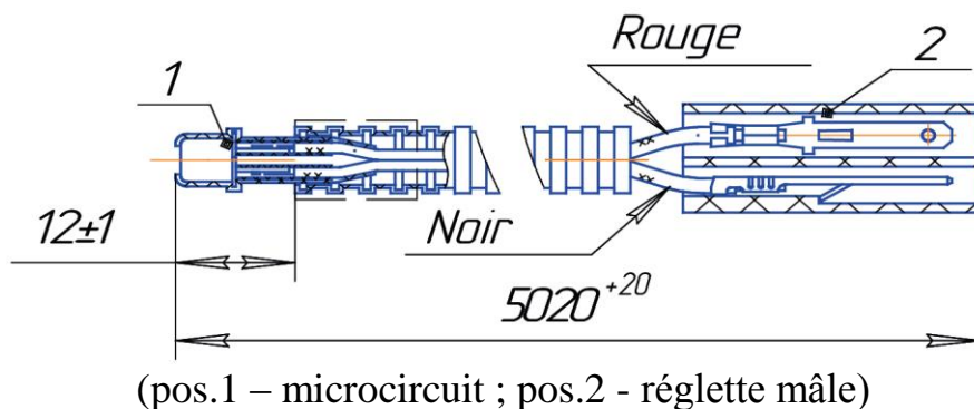
Fig.18 - Capteur de cabine
