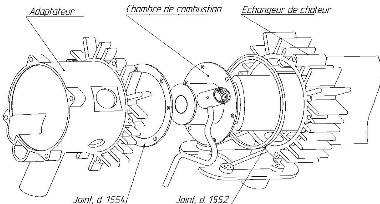
Fig.13 – Schéma d'installation de la chambre de combustion dans PLANAR-44D
