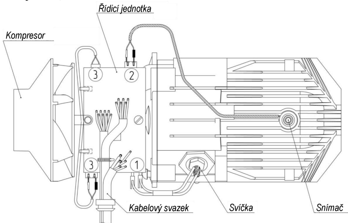
Obr. 2 - Ohřívač.
