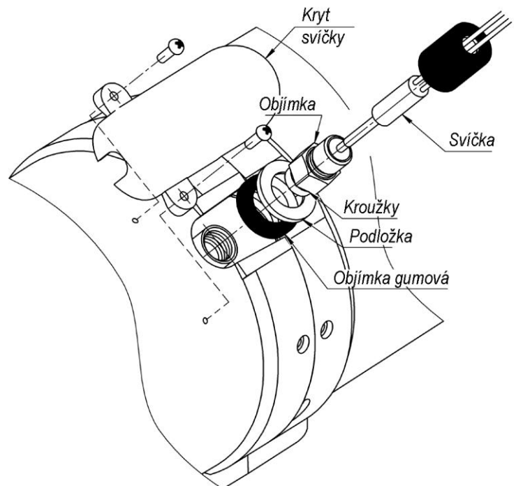
Obr. 4 - Svíčka s montážní sadou.
