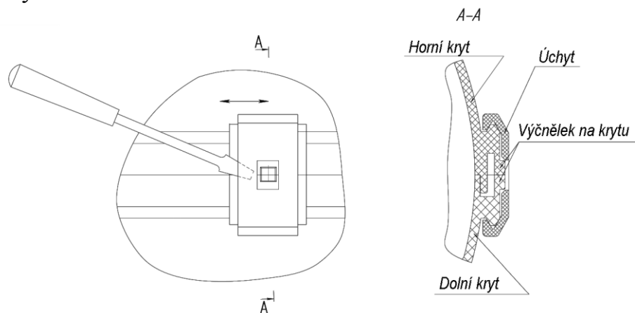
Obrázek 1 - Demontáž háčku z krytu ohřívače.
